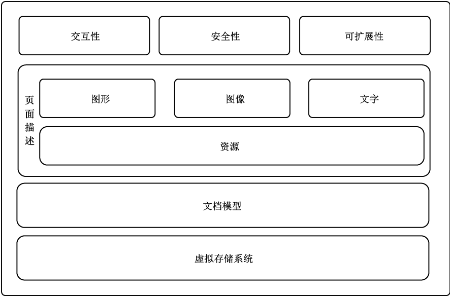
图 2 OFD 格式框架
